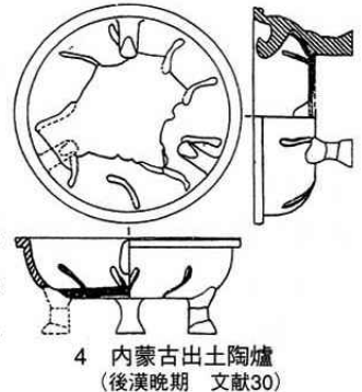
第18図 後漢の爐 1・4 1:8 2・3 1:6
