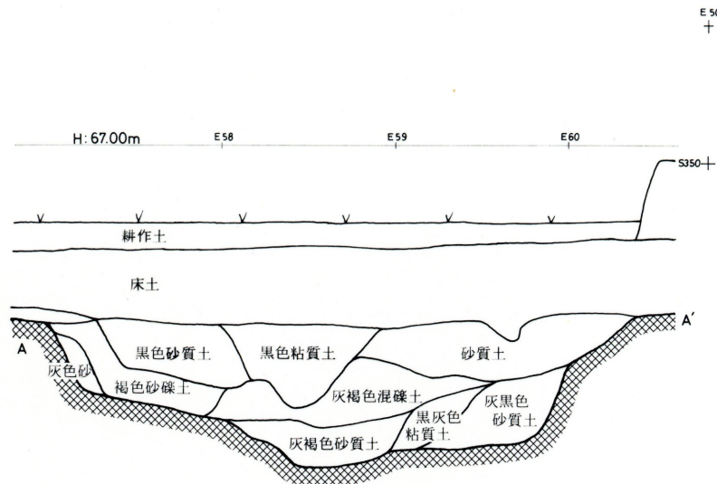
AA'断面土層図 1:40
