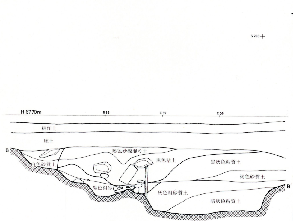
BB'断面土層図 1:40
