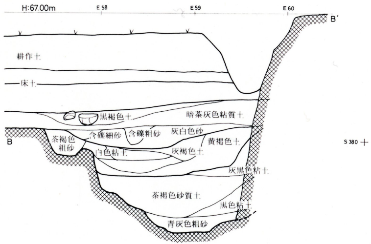
BB'断面土層図 1:40
