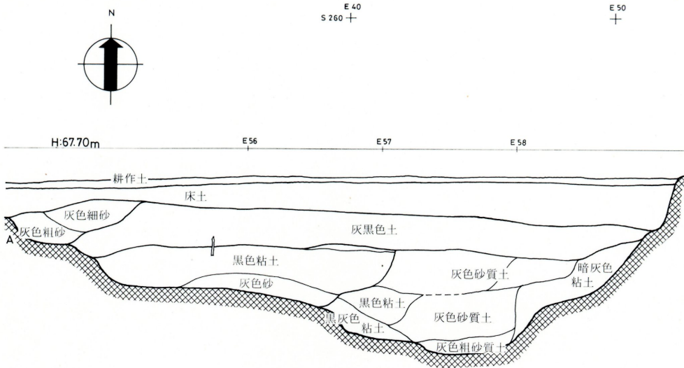
AA'断面土層図 1:40
