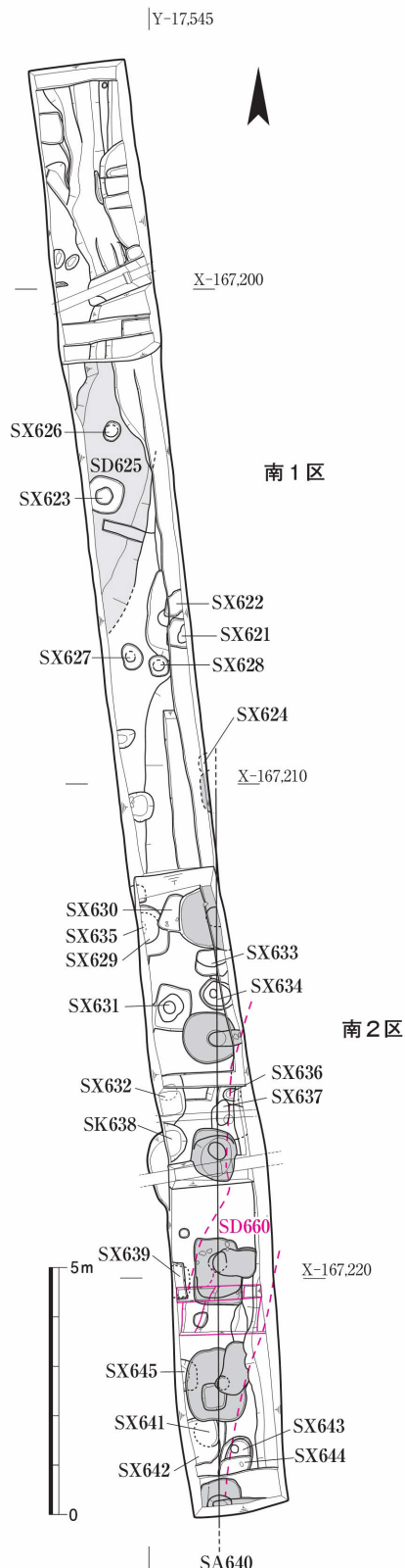
図115 南区遺構図 1:150
