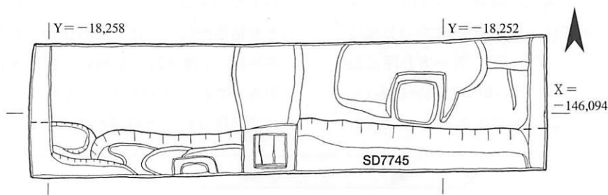
図83 第303-5次調査遺構図 1:80
