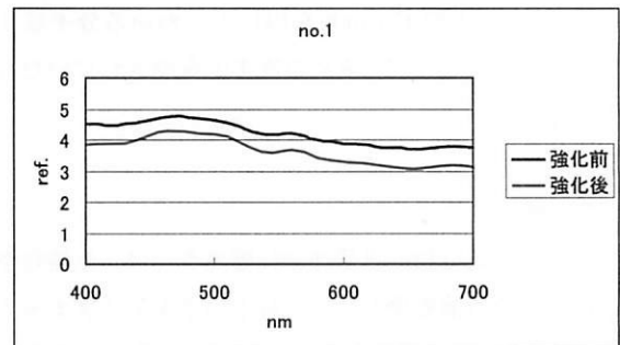
分光反射率図 (アクリル樹脂強化前後を示す)
