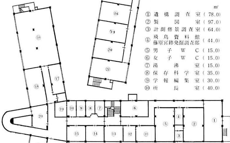
3階平面図
