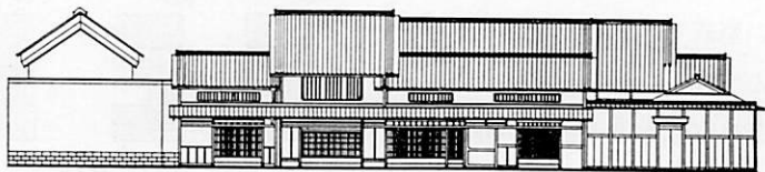
下御所町M家平面・立面図
