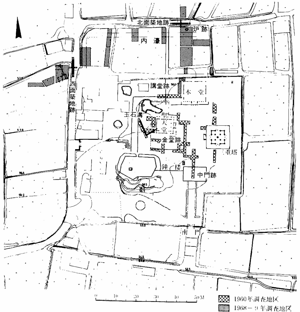
第1図 法起寺旧境内地形実測図
