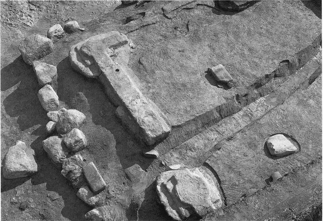
写真13 山田寺回廊東北隅扉口詳細
