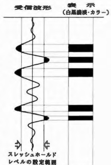
*23 受信波形とそれの表示
