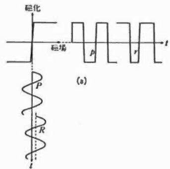
＊19 フラックスゲート型 磁力計の原理
