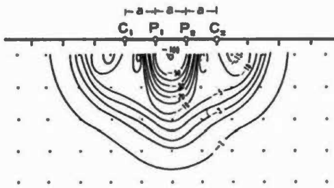
等間隔 CPPC 法 (ウェンナー法) 感度分布
