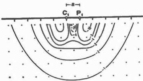
2極法感度分布
