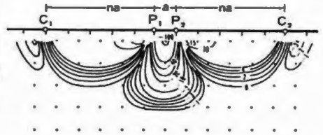
シュランベルジャー法感度分布
