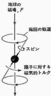
＊18 プロトン磁力計の原理
