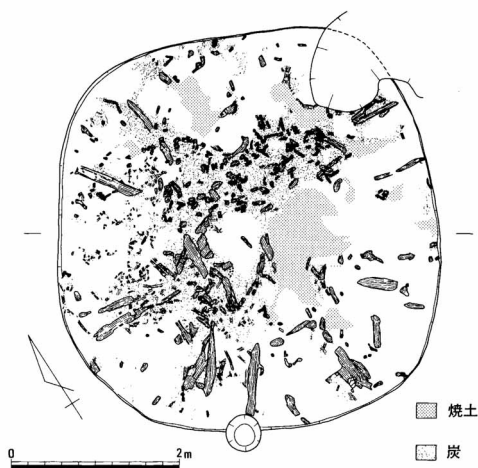
図64 焼失竪穴建物の一例 （岡山県教育委員会 1998 『窪木遺跡2』より）
