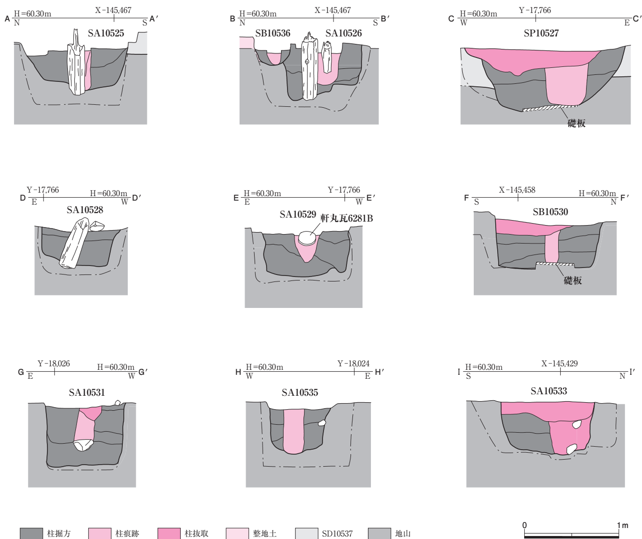
図274 第533次調査区柱穴断面図 1:40
