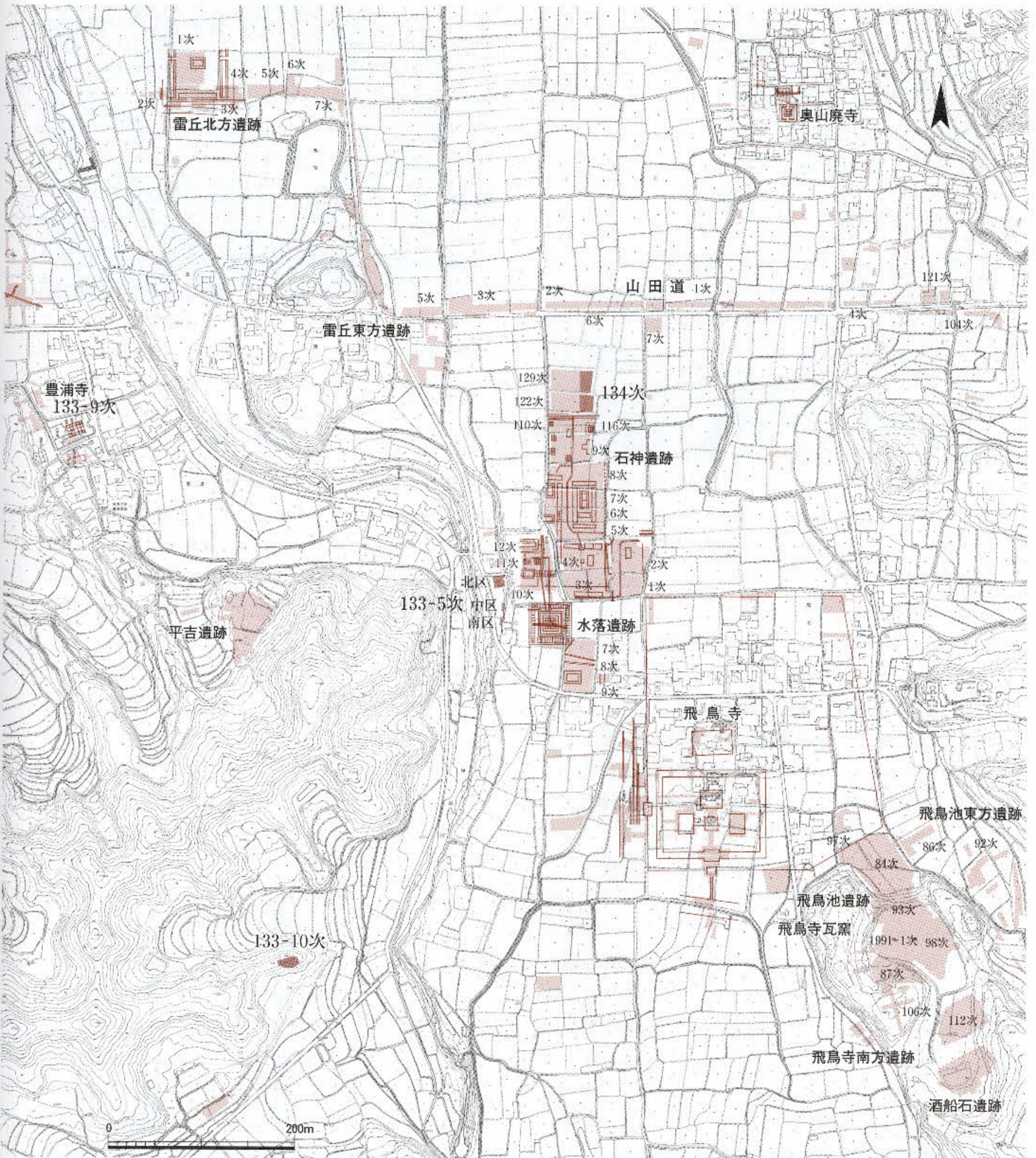
図97 飛鳥地域発掘調査位置図 1:6000
