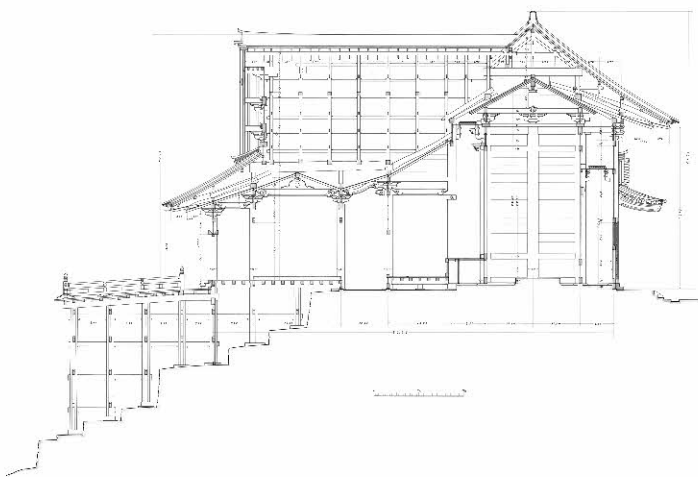
図B5 奥行方向の断面図 1:500
