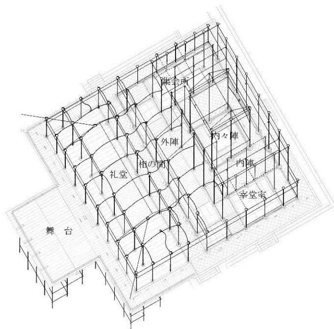
図B6 本堂架構図
