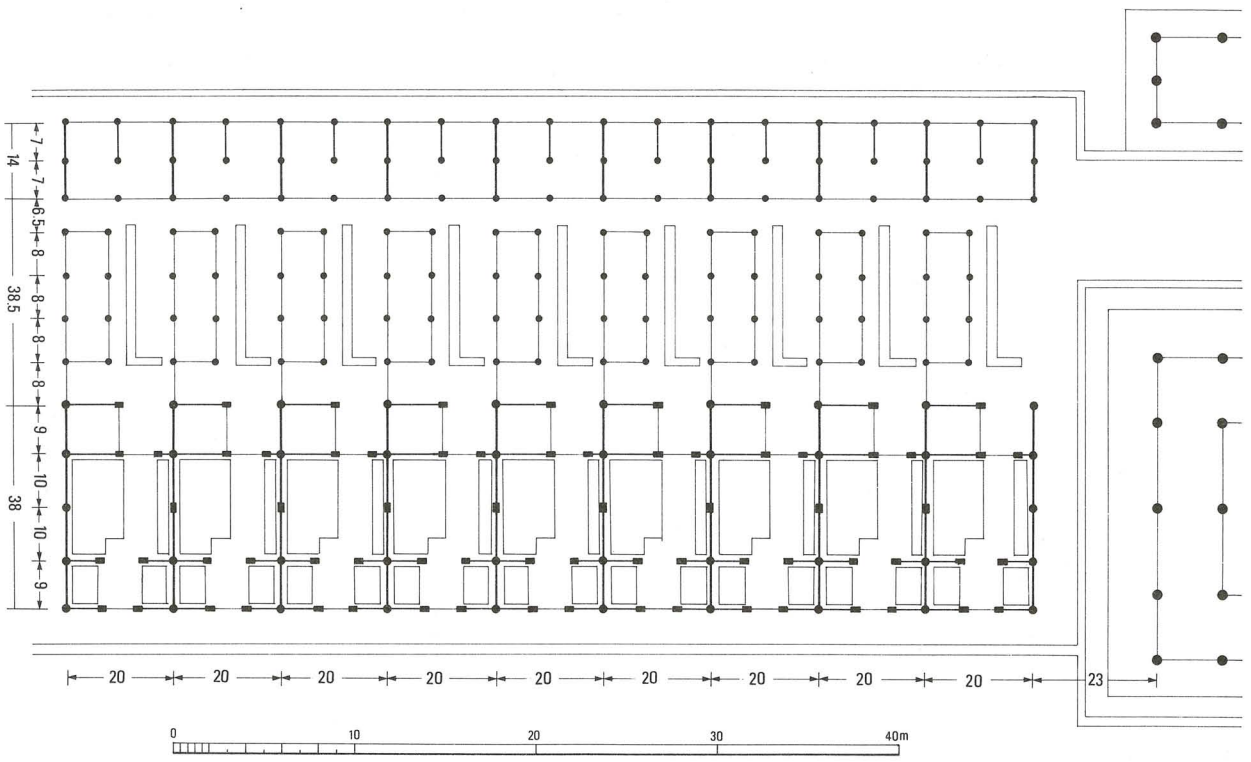
西僧房平面模式図
