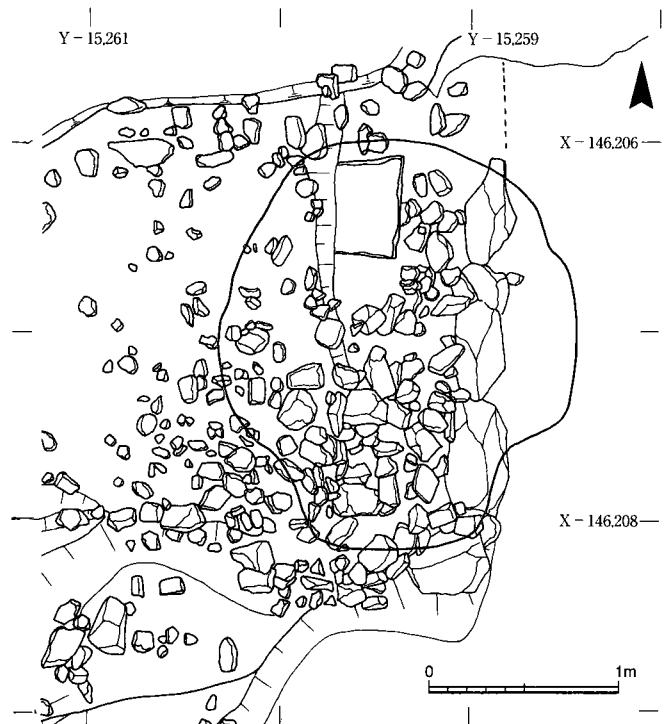
図160 SX8464とSE8465 1:40
