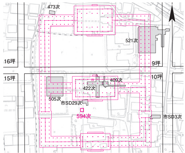
図270 第594次調査区位置図 1:2000
