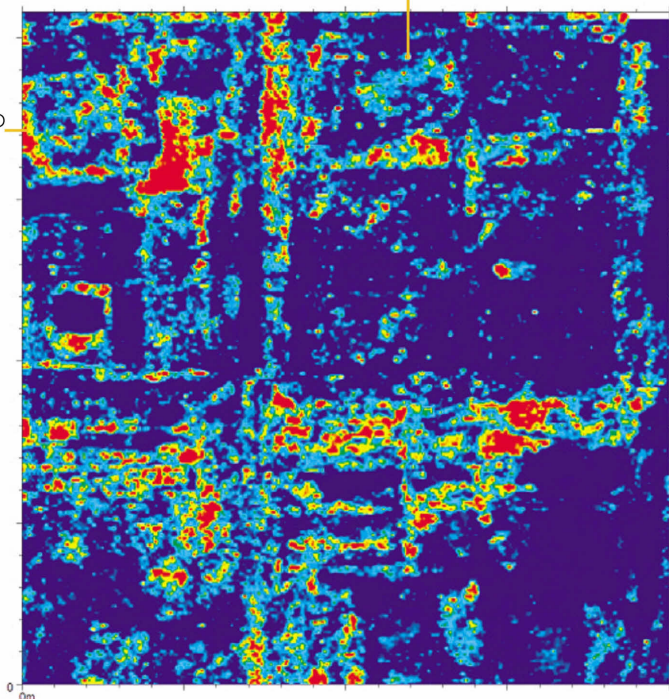
③地中レーダーによる探査成果（やや浅い部分）
