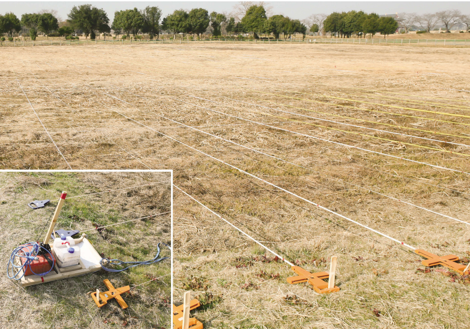
①探査のために張り巡らせた基準線と地面を這わすための櫛 くし にセットした地中レーダー(左下写真)
