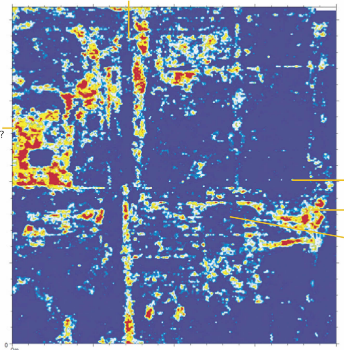
④地中レーダーによる探査成果（やや深い部分）
