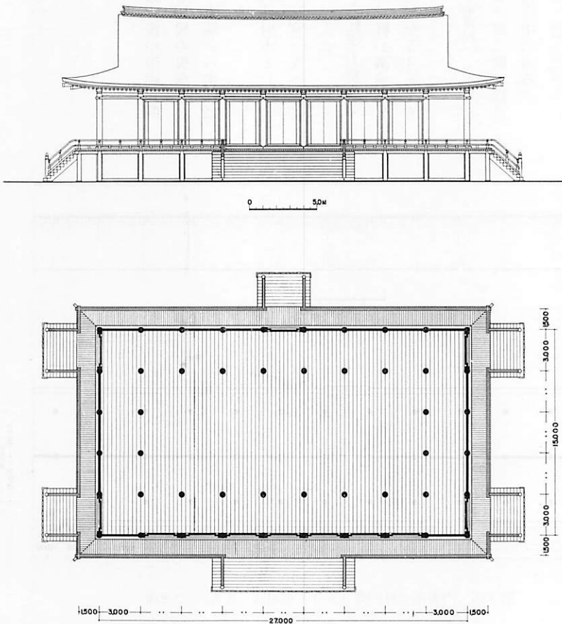
第2図 内裏正殿復原図 正面および平面
