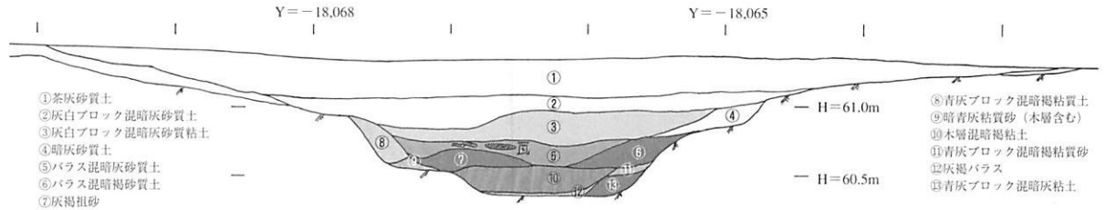
図5 東一坊大路西側溝SD4951断面図(②以下が下層堆積土) 1:50
