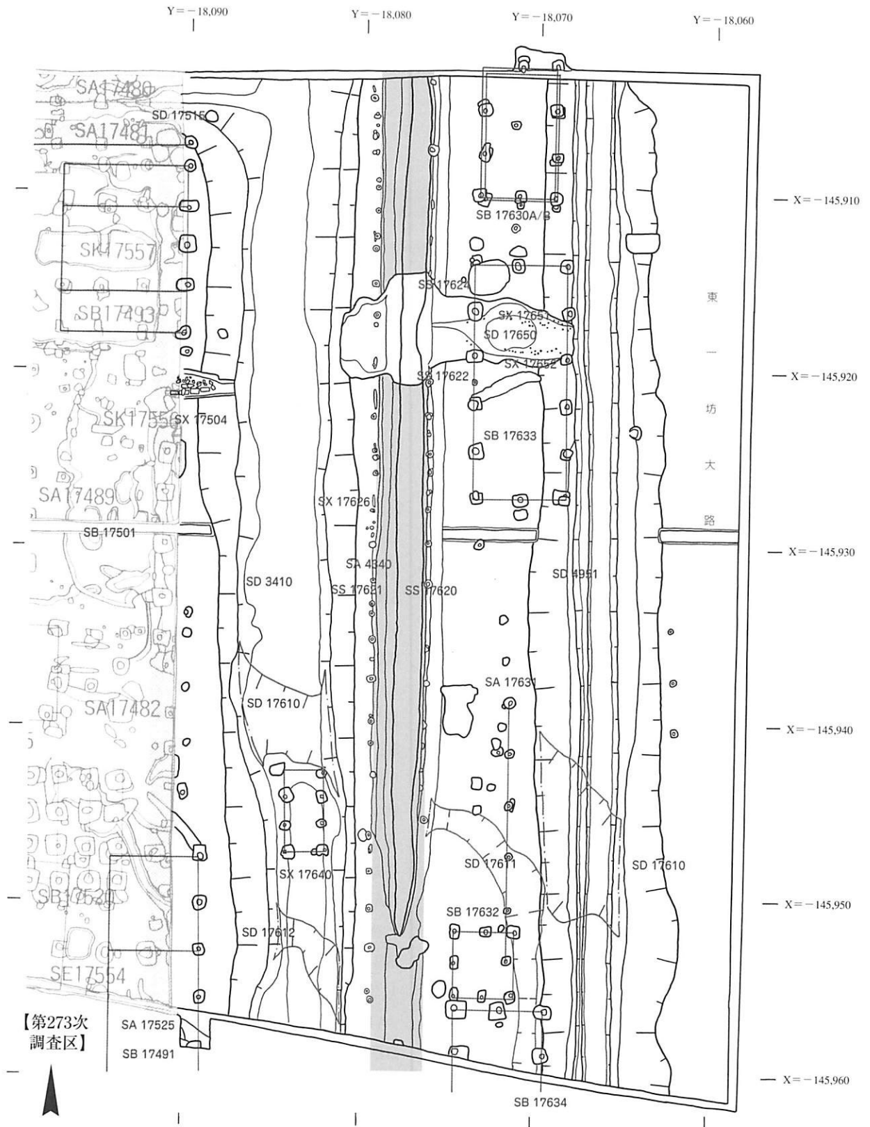
図3 第274次調査 遺構平面図 1:300
