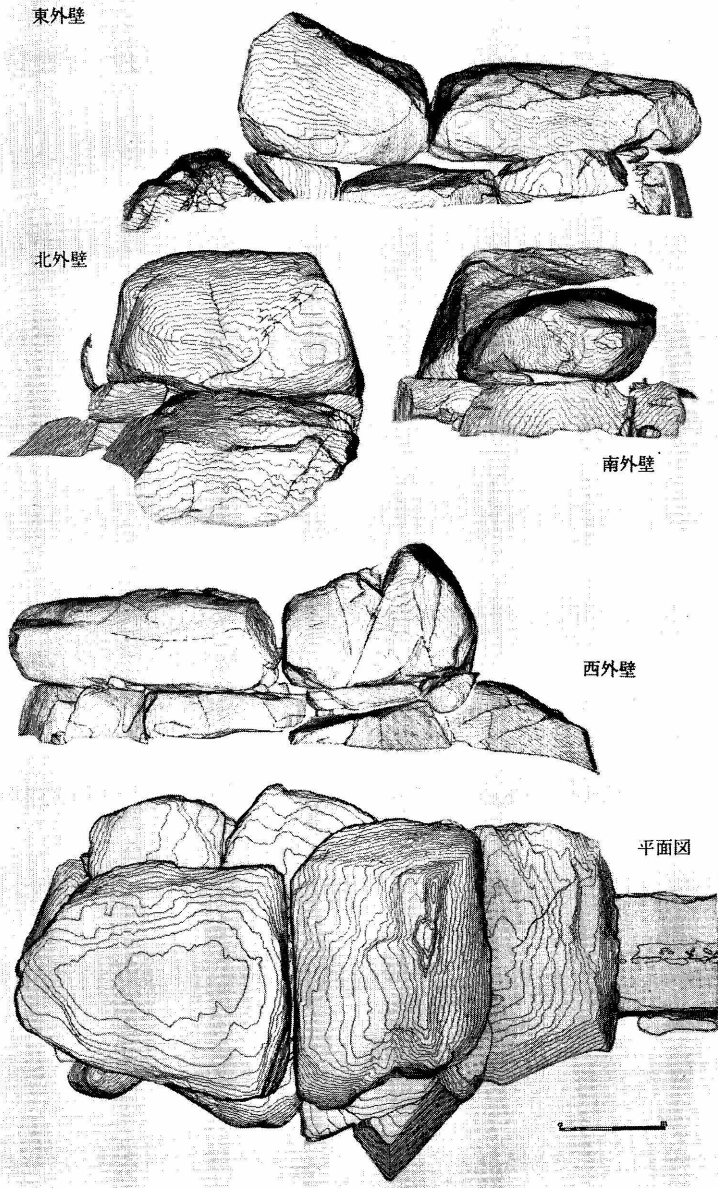
第2図 石舞台実測図
