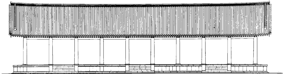
正面図
