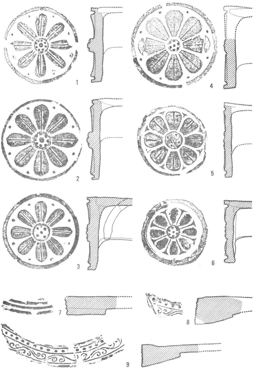
軒瓦実測図 (1/4)
