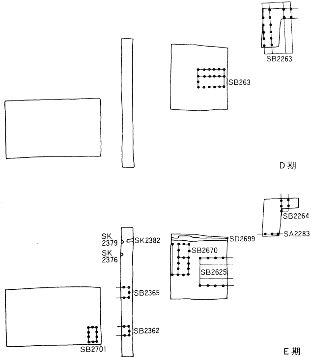
fig. 24 十三坪建物配置変遷図(2)
