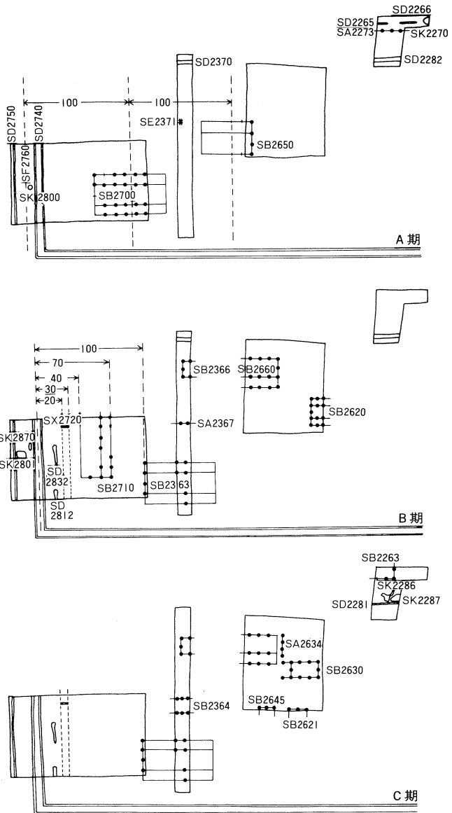
fig. 23 十三坪建物配置変遷図(1)
