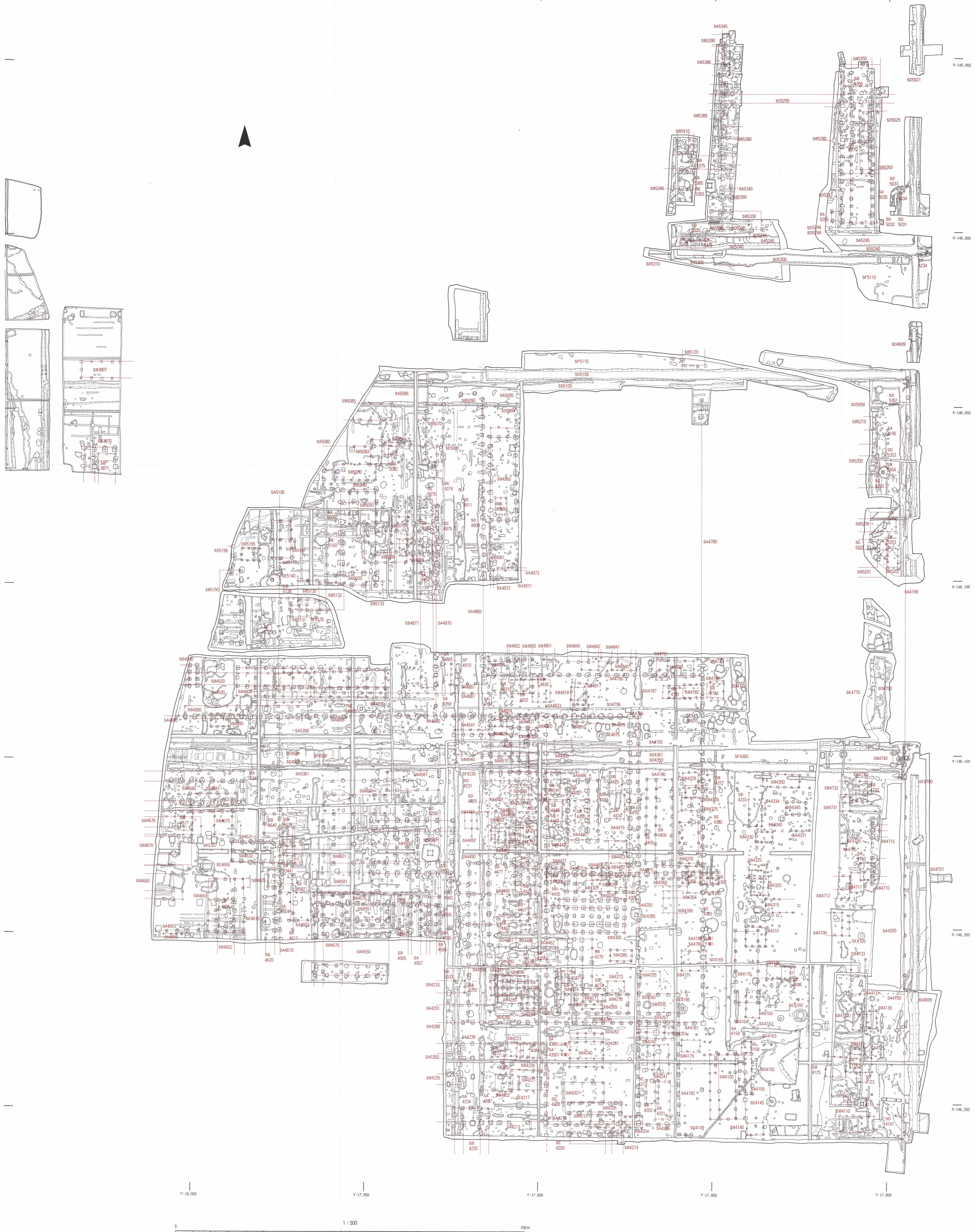
付図1 平城京左京二条二坊五坪、三条二坊一・二・七・八坪遺構配置図
