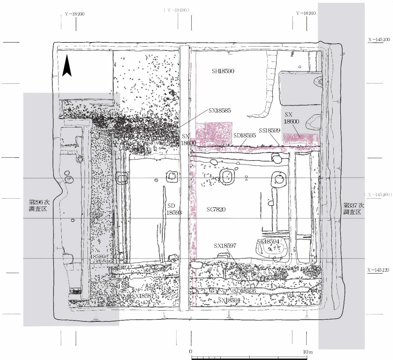
図149 第360次調査遺構平面図 1:200
