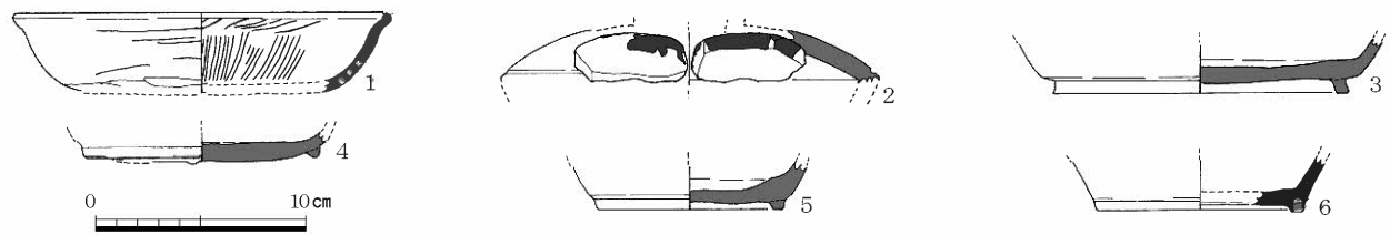
図58 第360次調査出土土器 1 : 4
