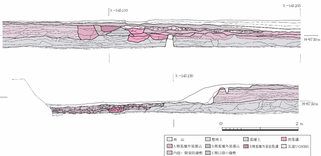
図150 調査区中央南北断面図(部分) 1:50
