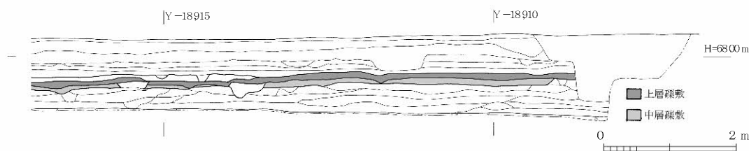
図51 内庭部東半東西断面図 1: 80
